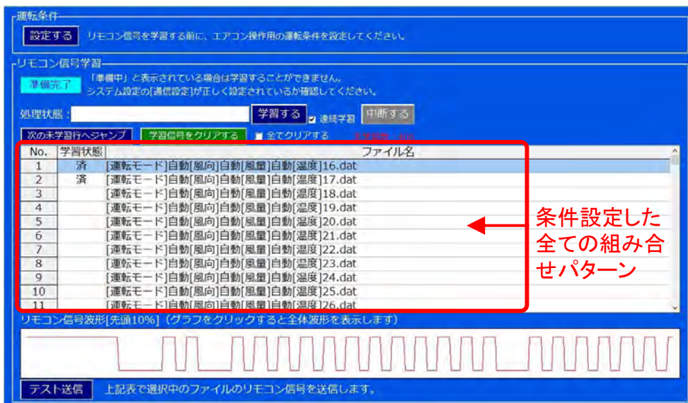
リモコン信号学習画面
